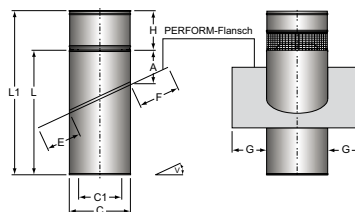
Standart A-Maß
