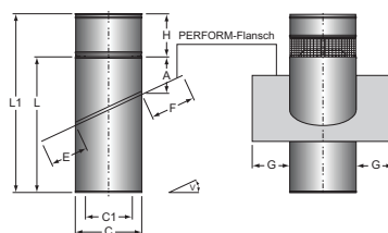
Standard A-Maß
